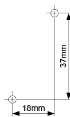
● 安装孔尺寸
